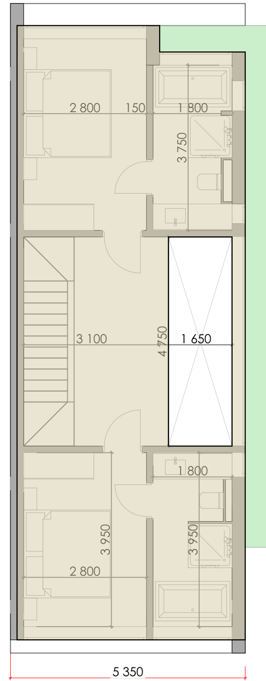
2 fl 64,48 м 2
