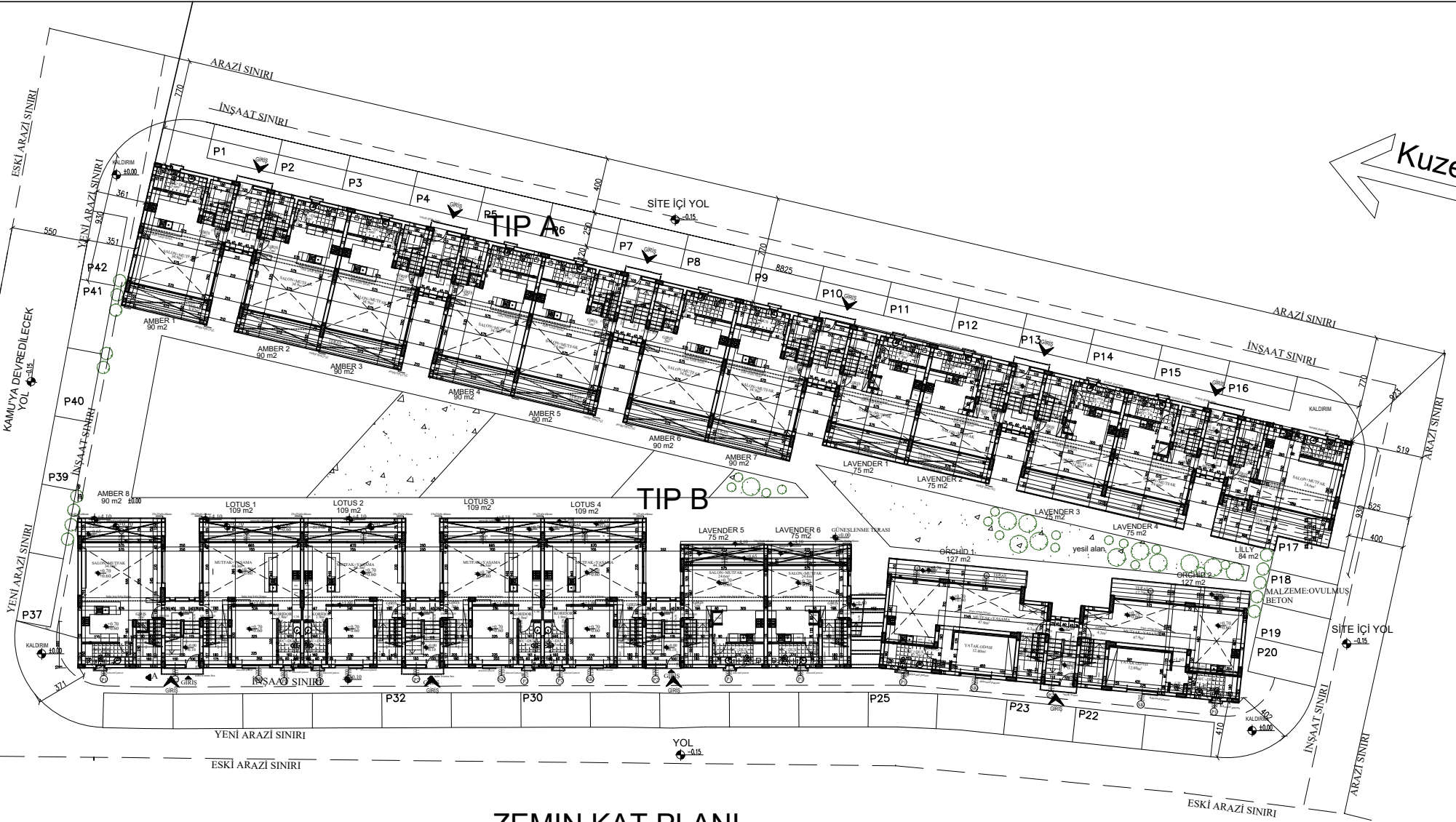
ZEMİN KAT PLANI
