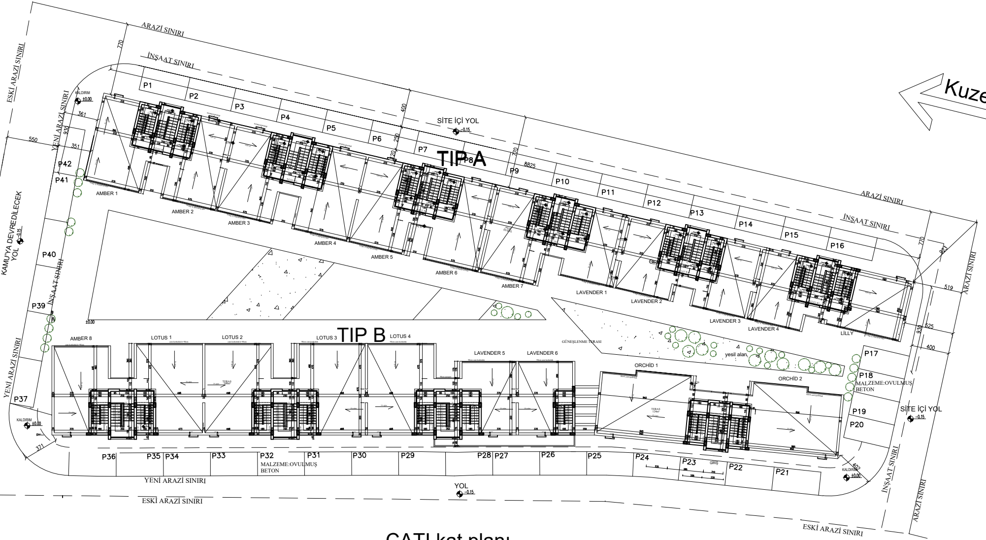
ÇATI kat planı
