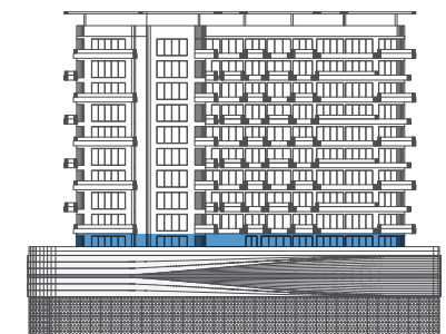
ELEVATION B
